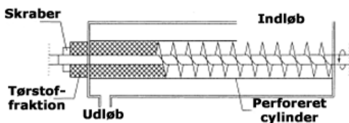
Figur 1. Principskitse af en skruepresse.
